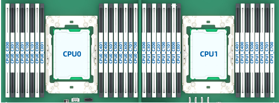
图 5-9 内存插槽位置
