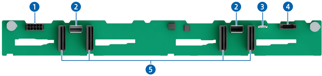
图 5-27 8 × 2.5 英寸 SAS/SATA/NVMe 硬盘背板
