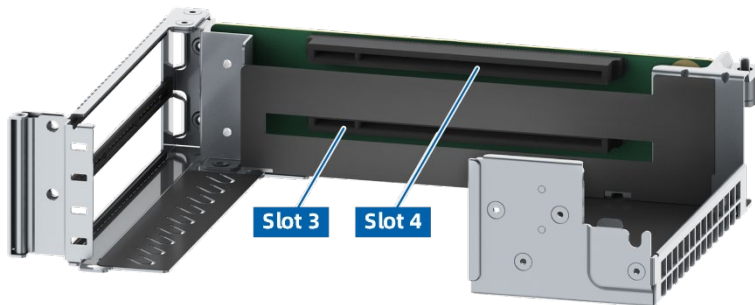
图 5-18 PCIe 转接卡模组 2
