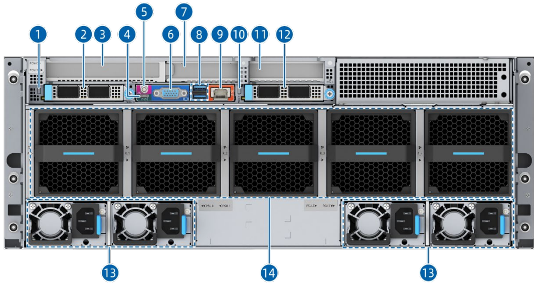
图 5-5 后面板外观
