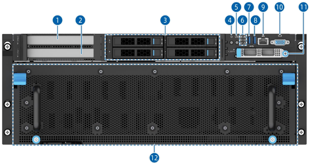
图 5-2 4 × 2.5 英寸硬盘配置前面板外观
