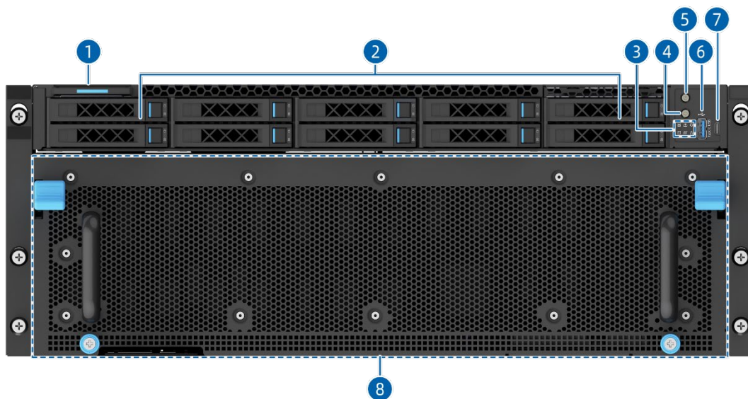
图 5-1 10 × 2.5 英寸硬盘配置前面板外观
