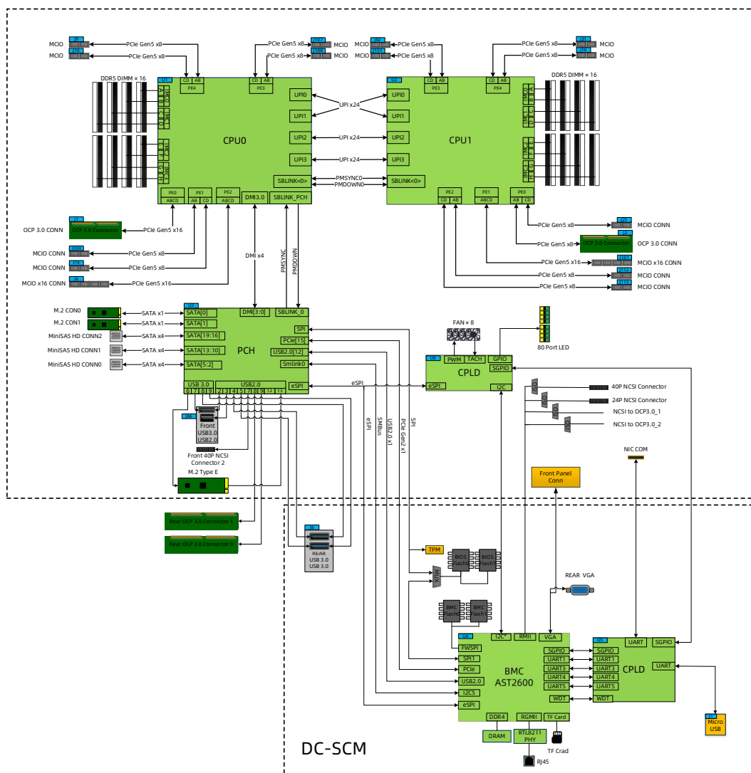
图 4-1 逻辑结构
