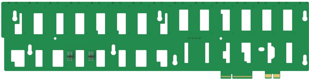
图 5-30 15 × 3.5 英寸 SAS/SATA 硬盘背板
