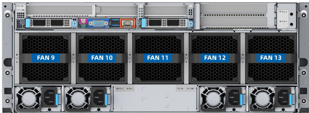
图 5-22 后置风扇模组的位置 (NF5476-M7-A0-R0-00)
