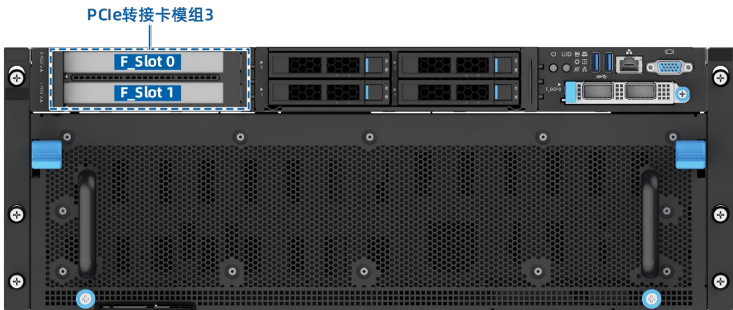
图 5-15 PCIe 插槽-前窗
