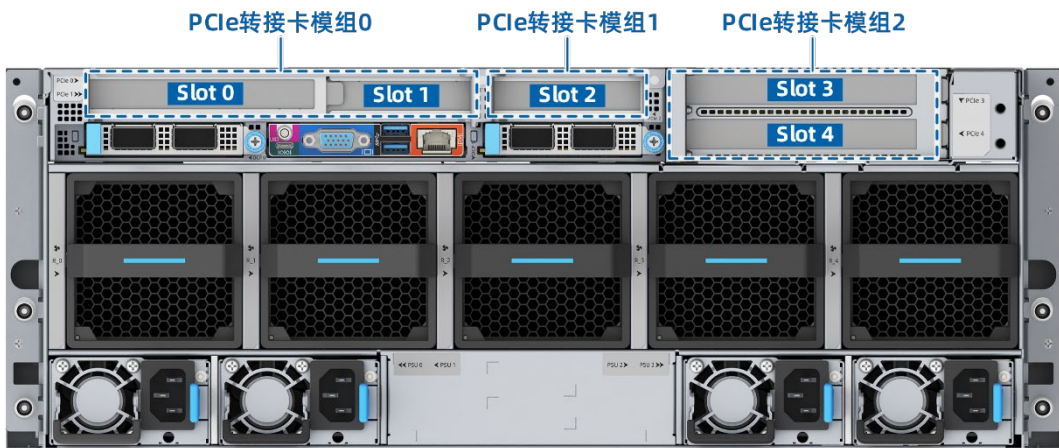
图 5-14 PCIe 插槽-后窗
