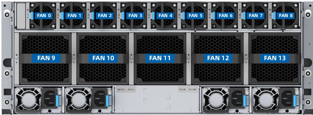
图 5-23 后置风扇模组的位置 (NF5476-M7-A0-F0-00)
