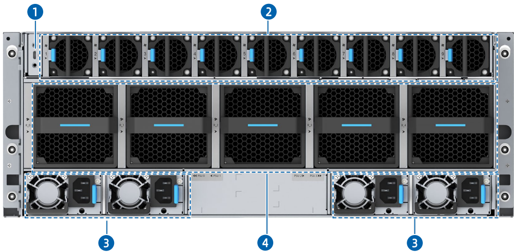
图 5-6 后面板外观
