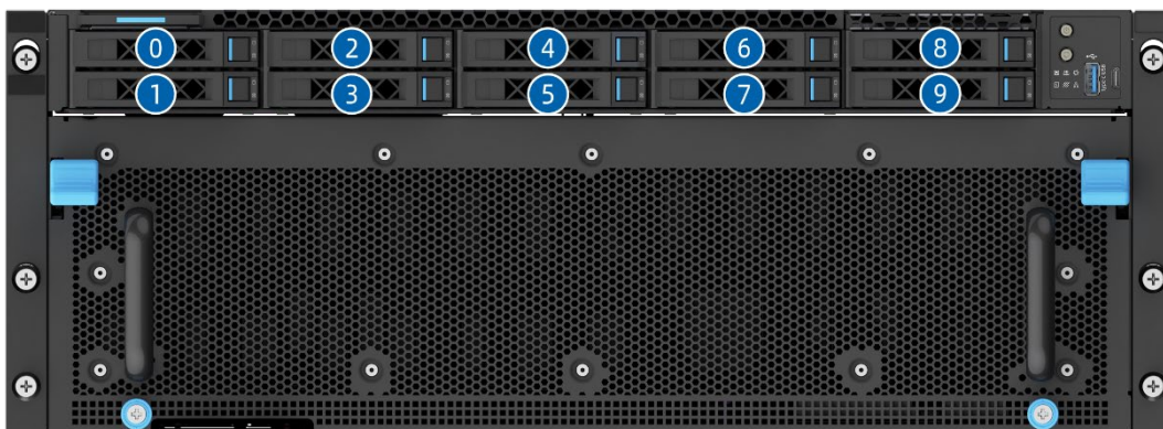
图 5-10 硬盘编号
