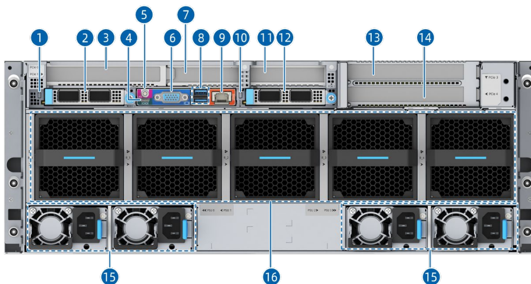
图 5-3 后面板外观
