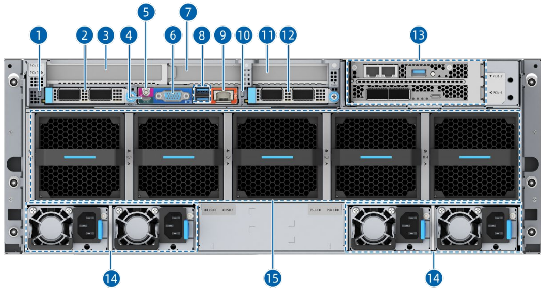
图 5-4 后面板外观
