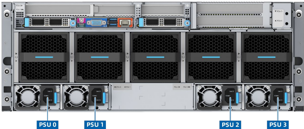
图 5-20 电源模块位置
