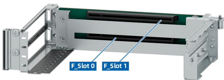
图 5-19 PCIe 转接卡模组 3
