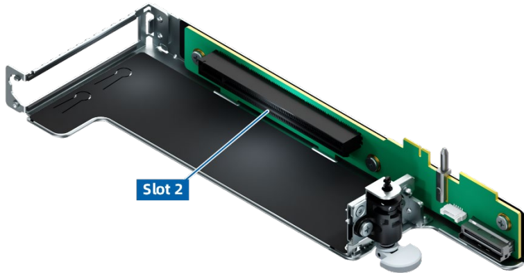
图 5-17 PCIe 转接卡模组 1
