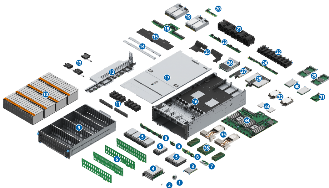
图 3-1 物理结构
