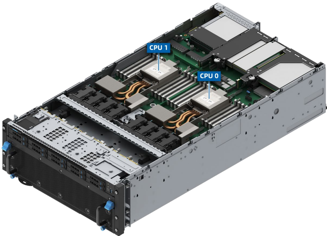
图 5-7 处理器位置
