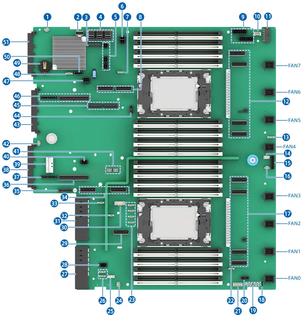
图 5-26 主板
