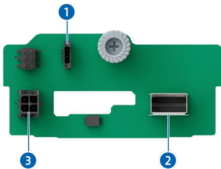
图 5-28 2 × 2.5 英寸 SAS/SATA 硬盘背板
