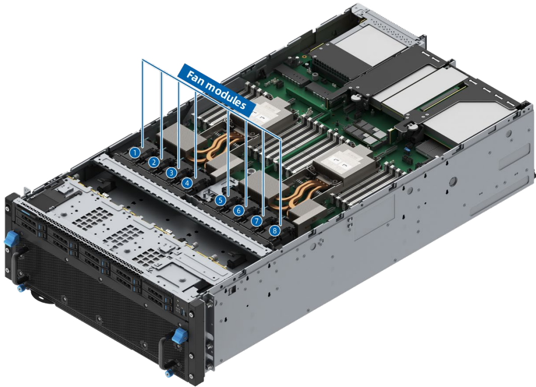
图 5-21 内置风扇模组的位置 (NF5476-M7-A0-R0-00)
