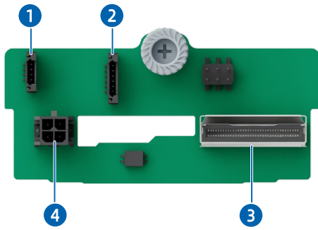
图 5-29 2 × 2.5 英寸 NVMe 硬盘背板
