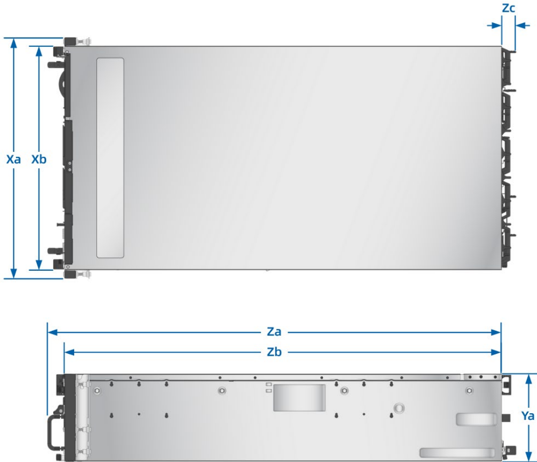
图 6-2 主机尺寸
