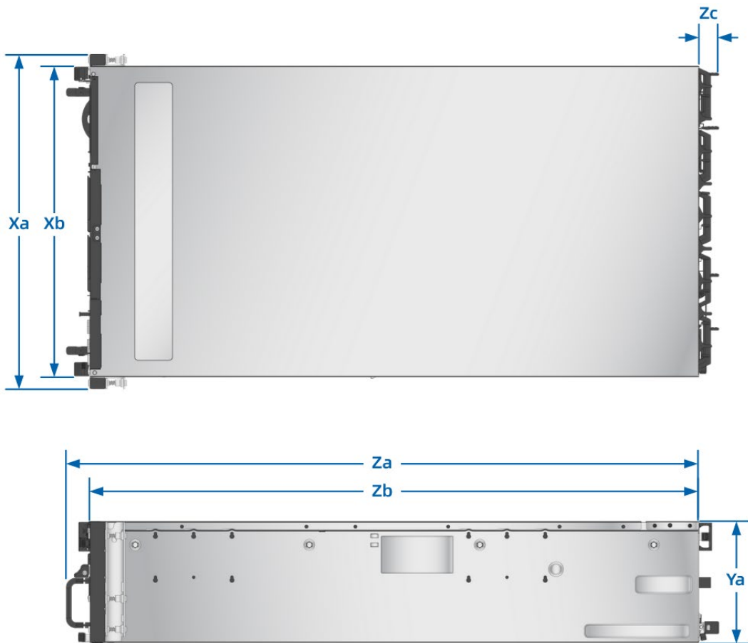
图 6-1 主机尺寸
