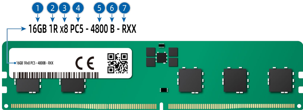
图 5-8 内存标识
